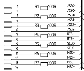
ST4 SMD-Siffleiste-7x2-RM2-180°
