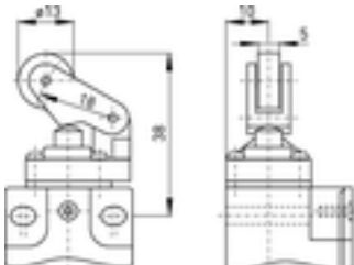
Kunststoff-Rollenhebel WH
