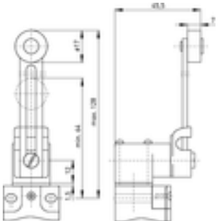
Stellbarer Drehhebel DS
