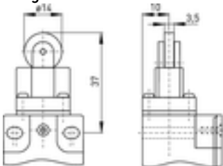
Langer Rollenstößel RL
