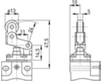
Kipphebel WHKM
