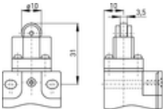
Rollenstößel R
