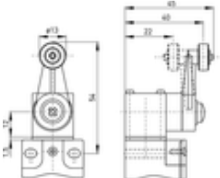
Drehhebel D
