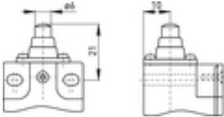
Stößel W
