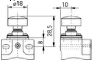
Kappe WK
