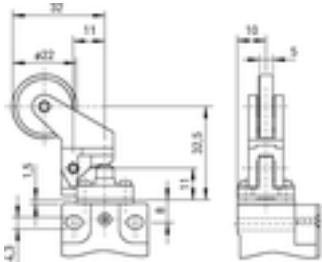
Kunststoff-Rollenhebel 4K
