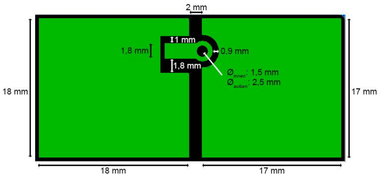
Abb. 2 - Platinenlayout
