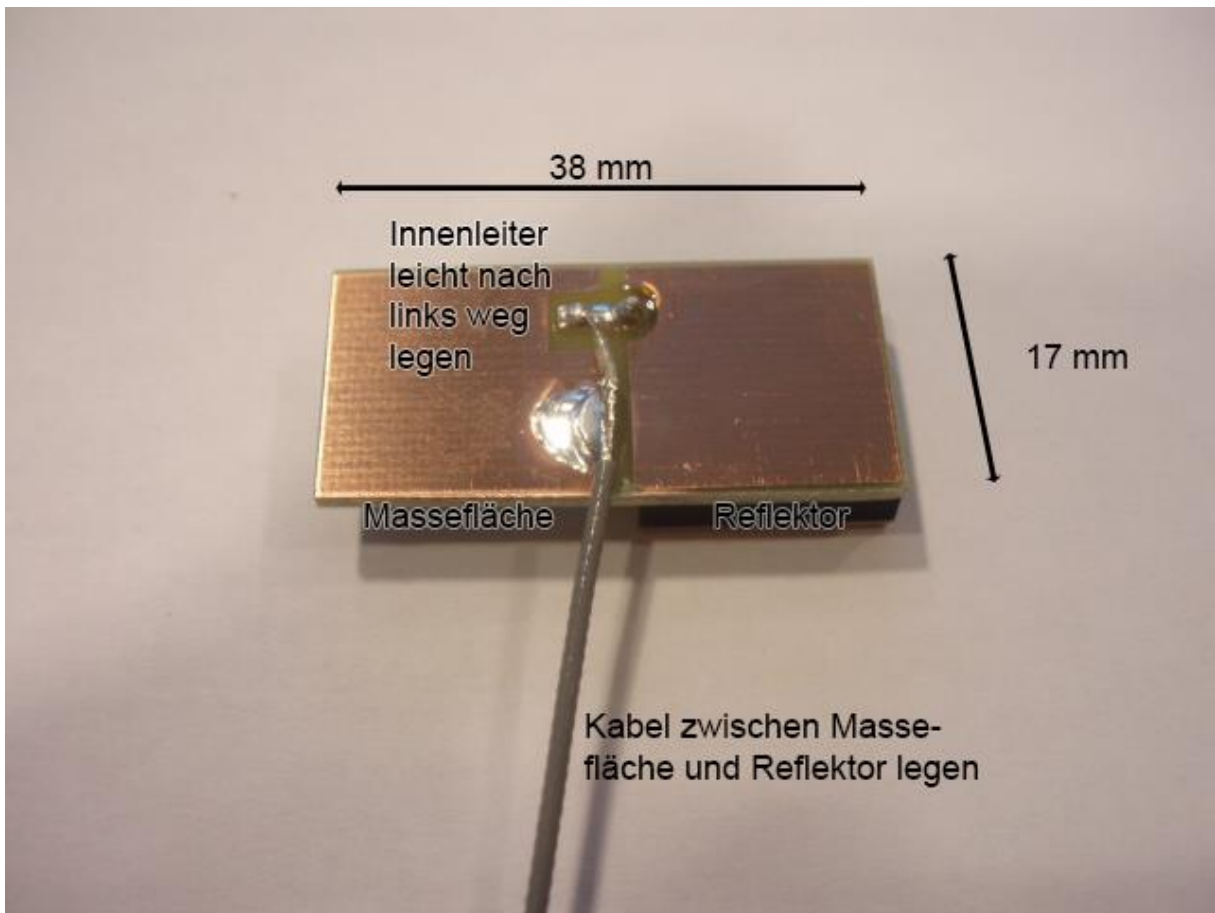
Abb. 1 - Board mit U.FL-Kabel
