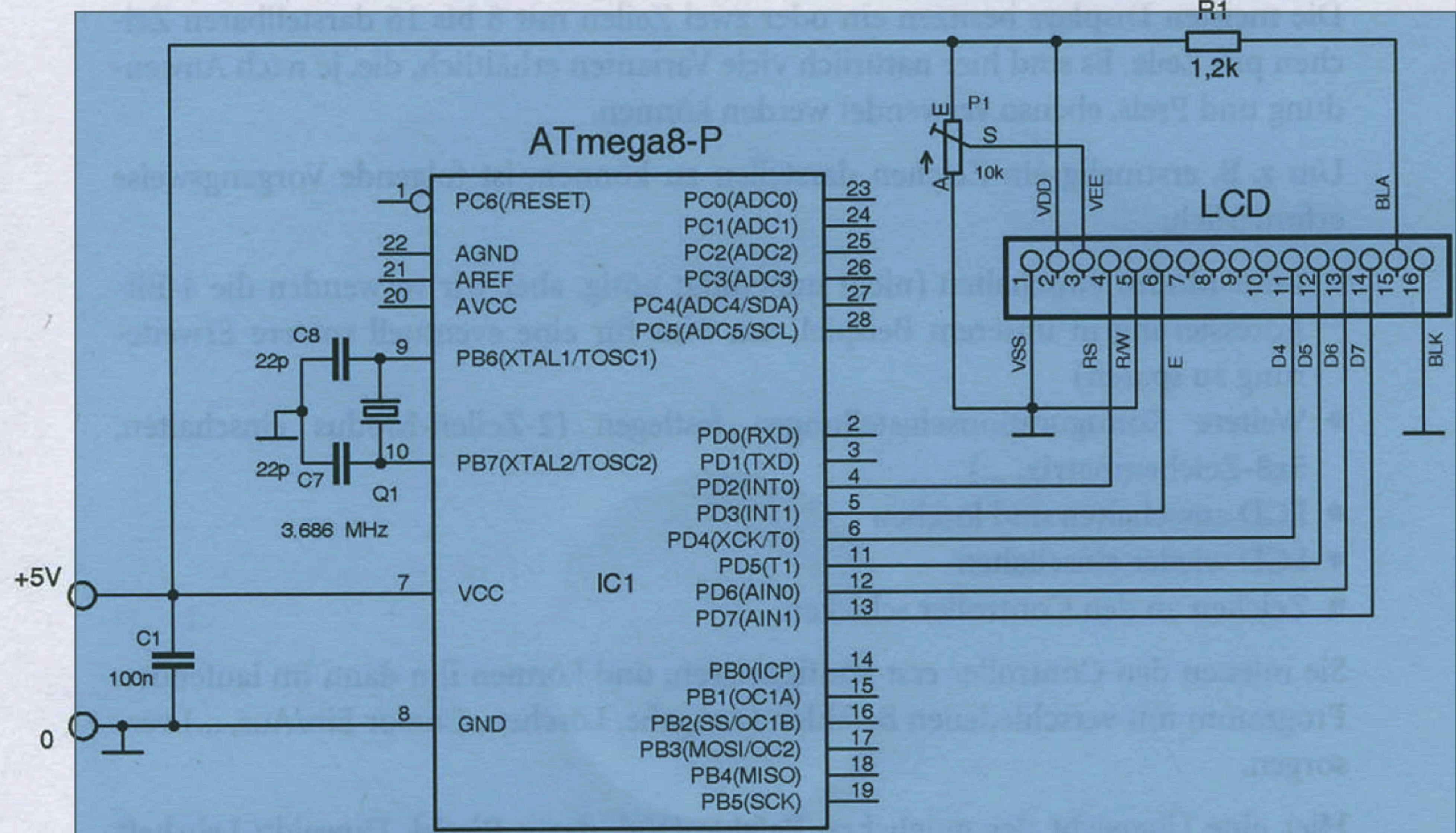
Abb. 5.3: Schaltung der LCD-Steuerung
