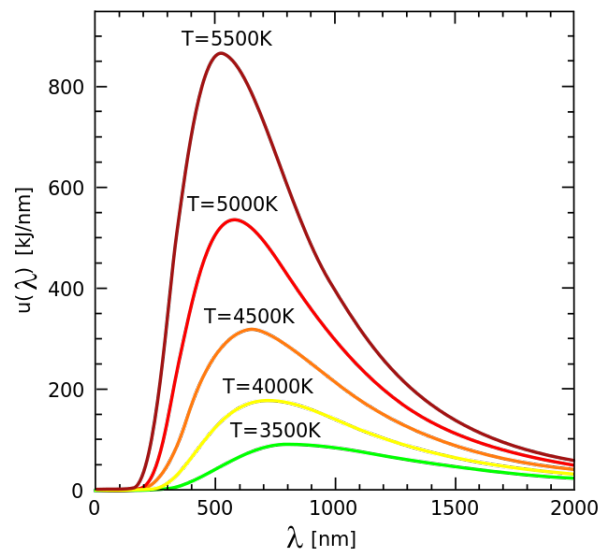
Abbildung 2: Spektrum des schwarzen Strahlers
