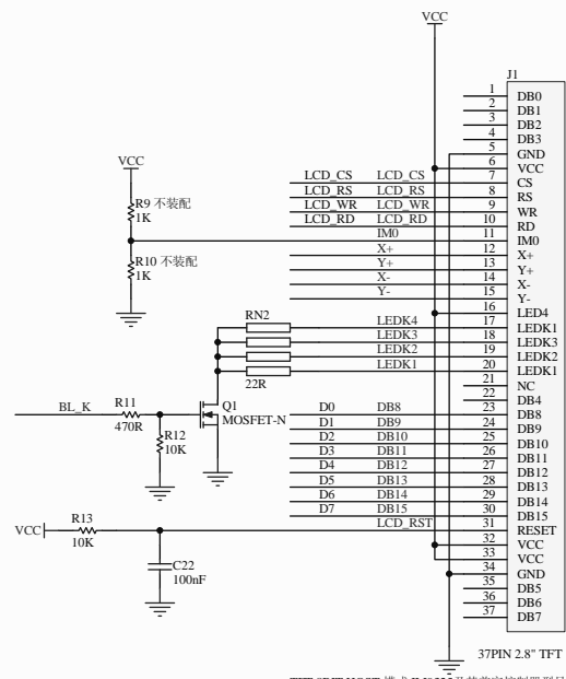
TFT 8BIT HOST 模式 ILI9325及其兼容控制器型号
