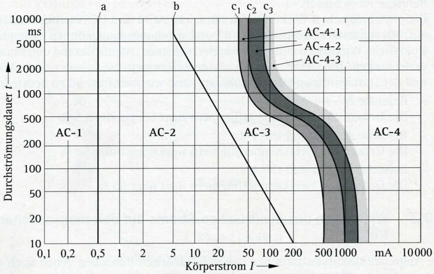
Wirkungsbereiche von Körperströmen bei Wechselstrom; Effektivwerte bei 15 Hz bis 100 Hz
