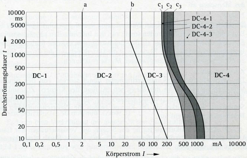
Wirkungsbereiche von Körperströmen bei Gleichstrom
