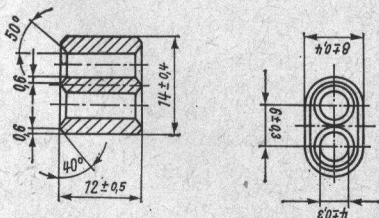
Bild 4 Mehrlochkerne aus Manifer
