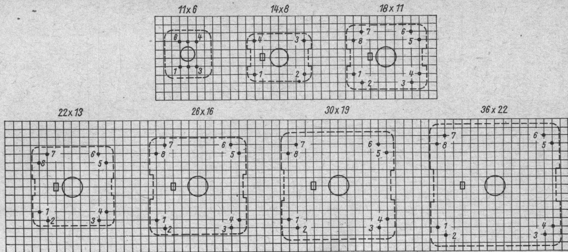
Bild 9 Rastermaße der Schalenkern-Armierungen für gedruckte Verdrahtungen
