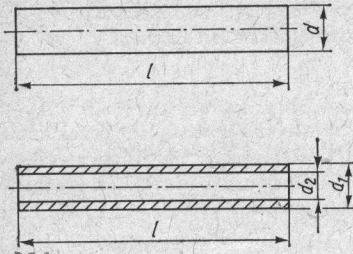
Bild 1a Zylinderkerne ohne Gewinde
