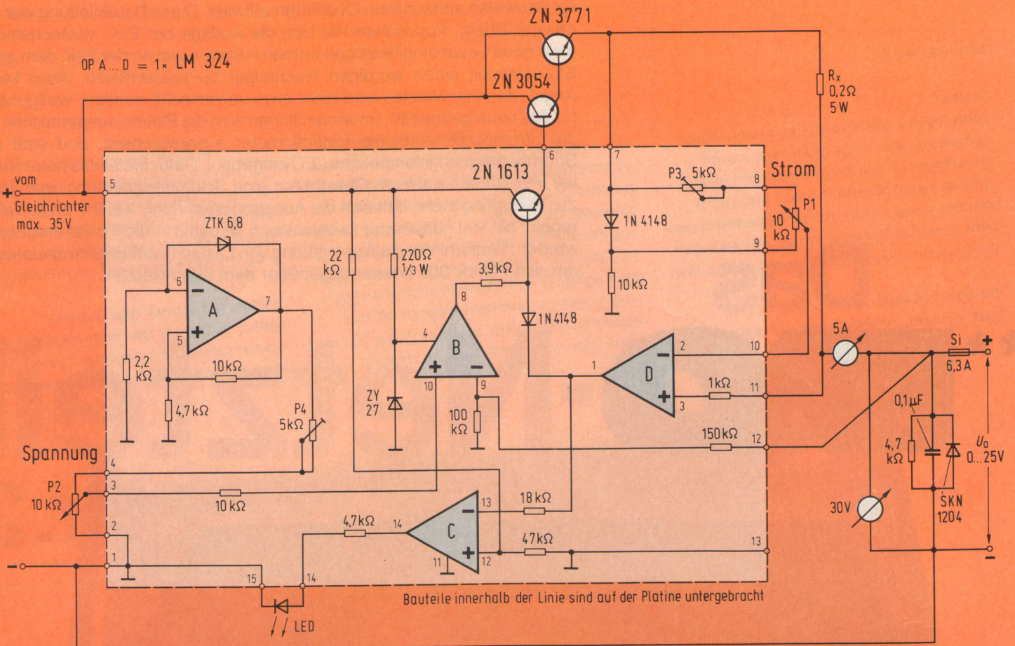
Bild 1: Die Schaltung des neuen Regelteiles für das ELO-Netzgerät Nr. 2.
