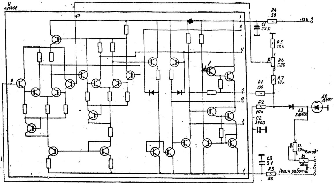
КАЛИБРАТОР Схема электрическая принципиальная И25.085.001Э3
