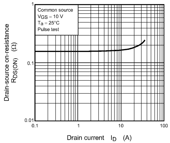
Fig. 8.6 R_{DS(ON)} - I_D
