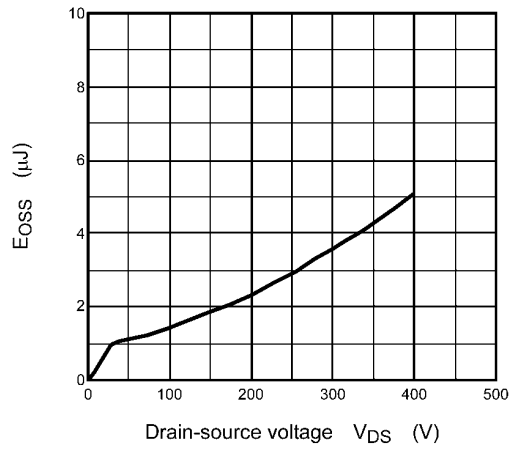
Fig. 8.10 E_{OSS} - V_{DS}
