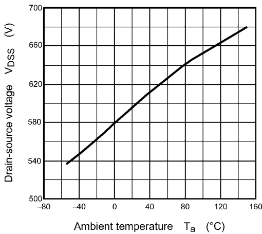
Fig. 8.5 V_{DS} - T_a
