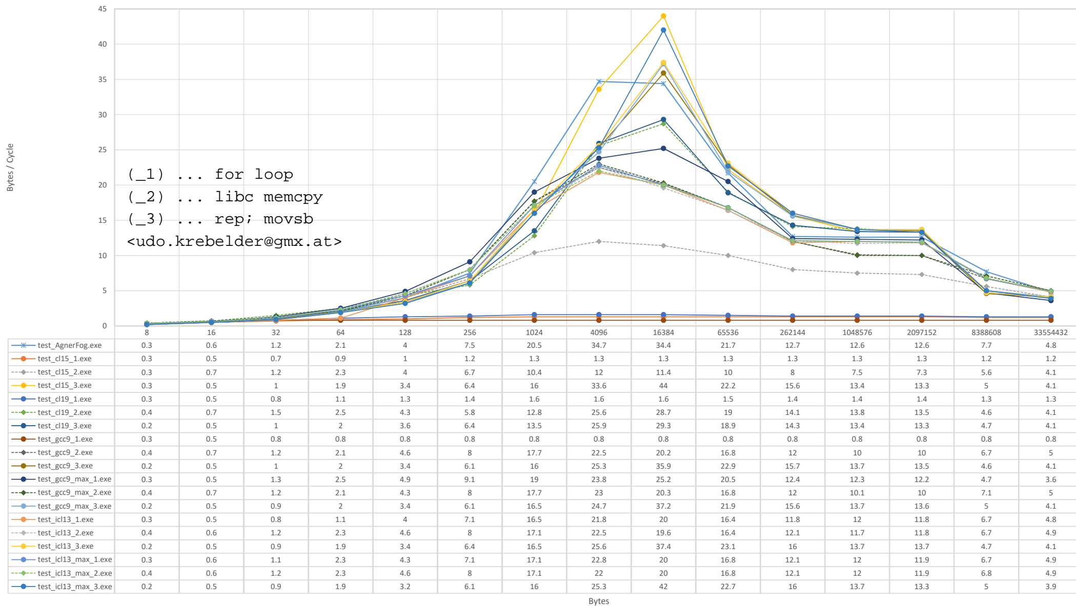
Memcpy Bytes/Cycle über Buffergröße
