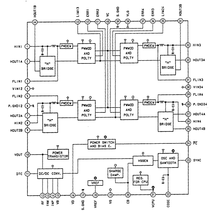
IC504 MPC1715
