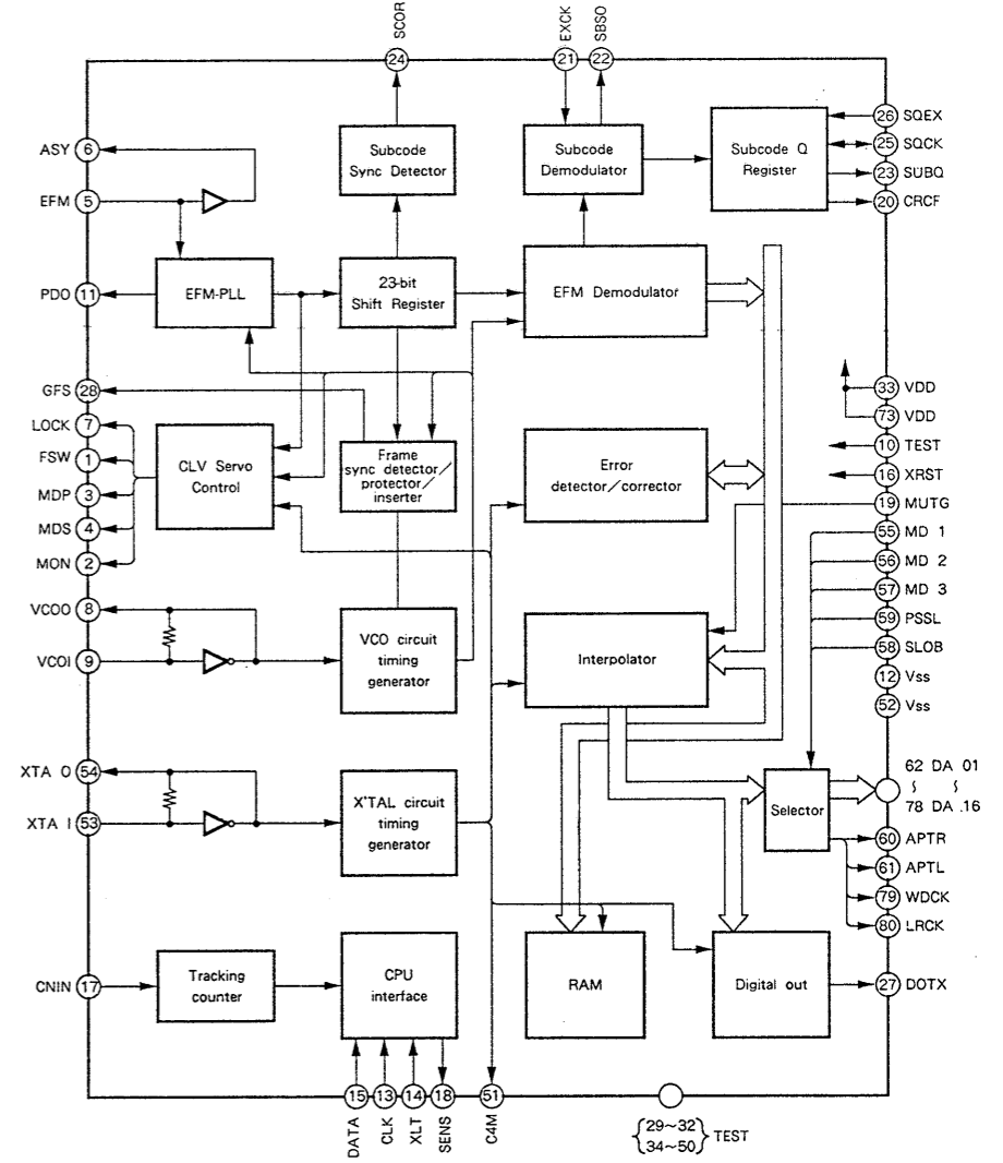
IC601 CXD1167Q
