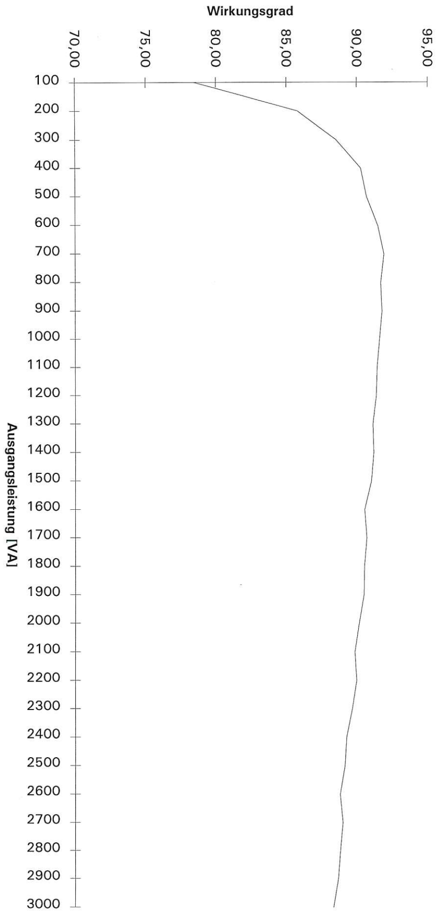
WRA30/24 Wirkungsgrad
