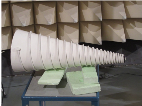
Antenne Rhode und Schwarz HUF-Z4, 200 – 1000MHz
