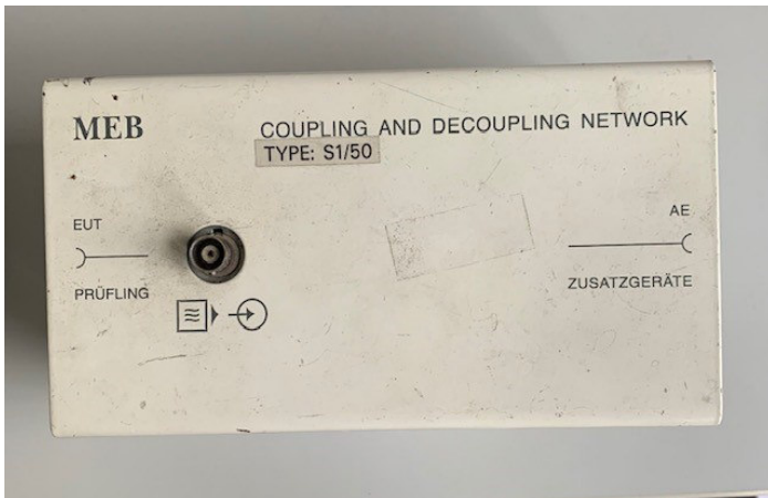
Koppelnetzwerk S1 50
