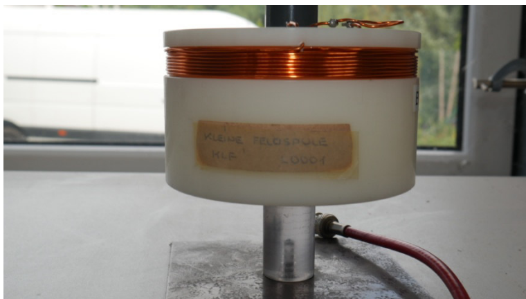
Kleine Feldspule EN 55103-1
