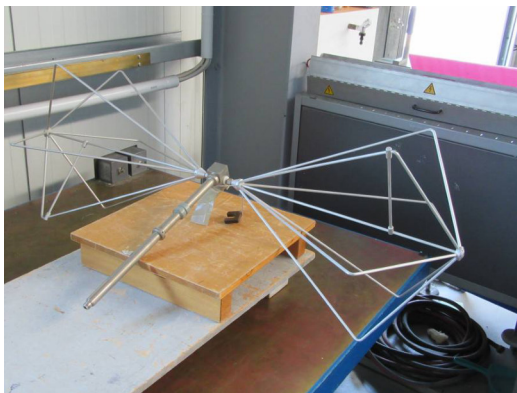
Antenne Schwarzbeck VHA 9103, 25 – 300MHz
